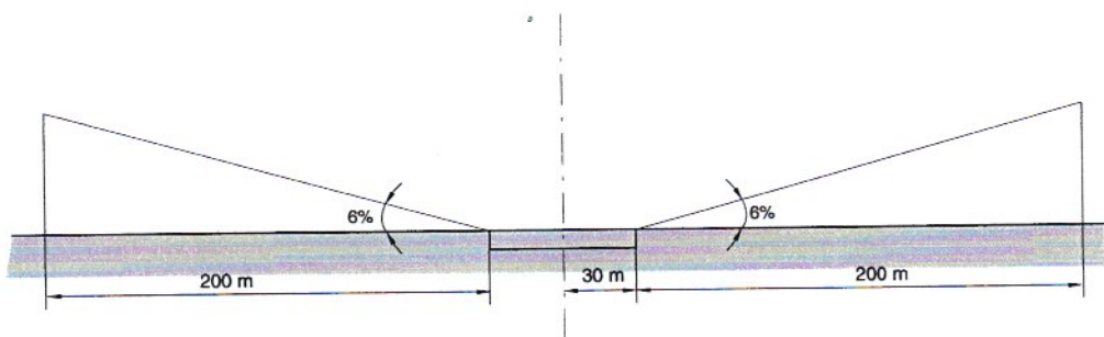
13-45 Dégagements pour une infrastructure de classe UA
