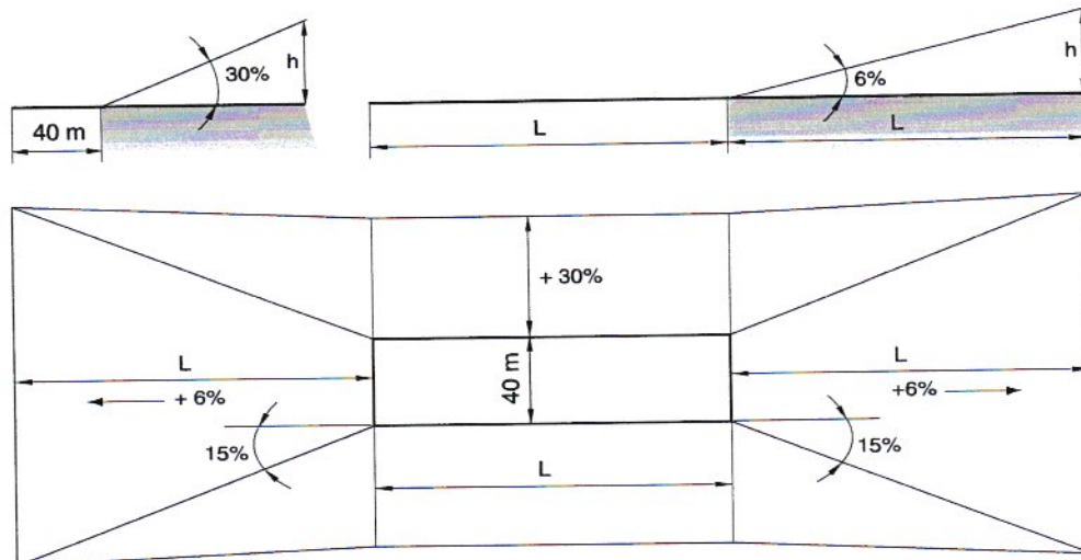
13-44 Dégagements pour les infrastructures de classe UB
